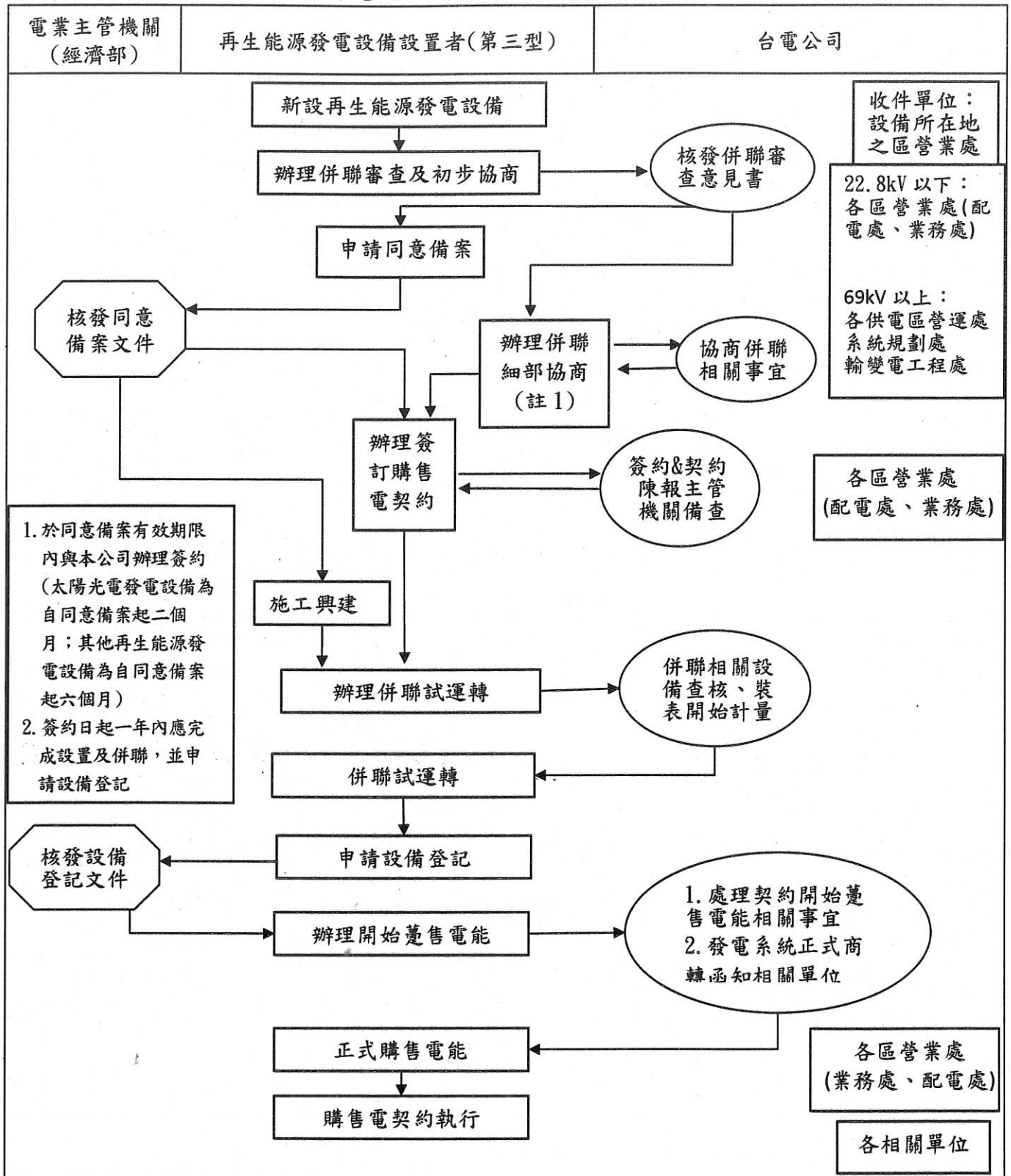
附圖 1 台電公司再生能源電能收購作業流程(第三型)
